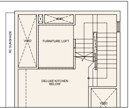
LOFT - PLAN
